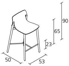
KAYAK STOOL / 051
